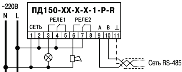
Рисунок Б.2 – Пример схемы подключения преобразователя с RS-485
